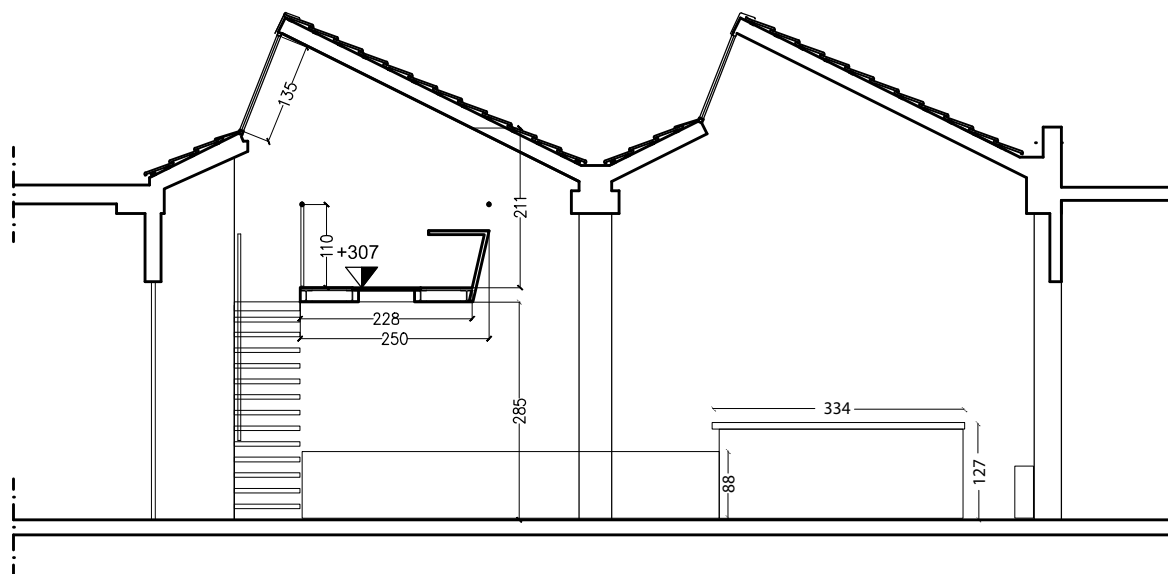
SEZIONE A-A
